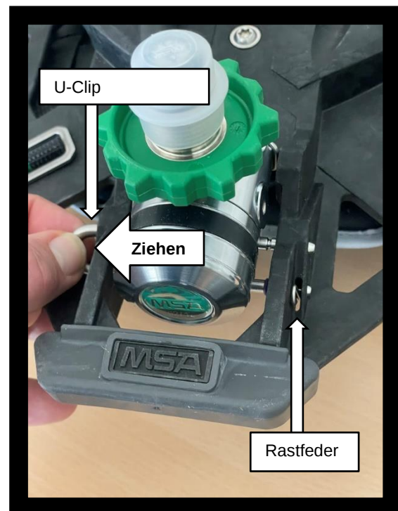
Abb. 4 – Funktionsprüfung U-Clip
